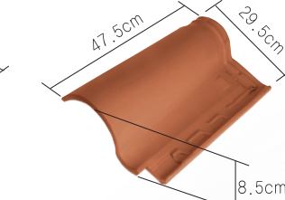
환기기와(TB-10) 4.10Kg
